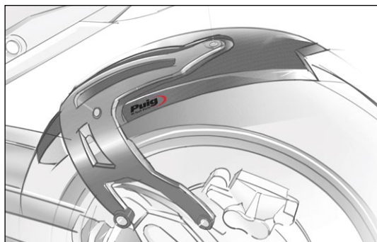
BMW R1200R 15'-18' (PART# 7682)
